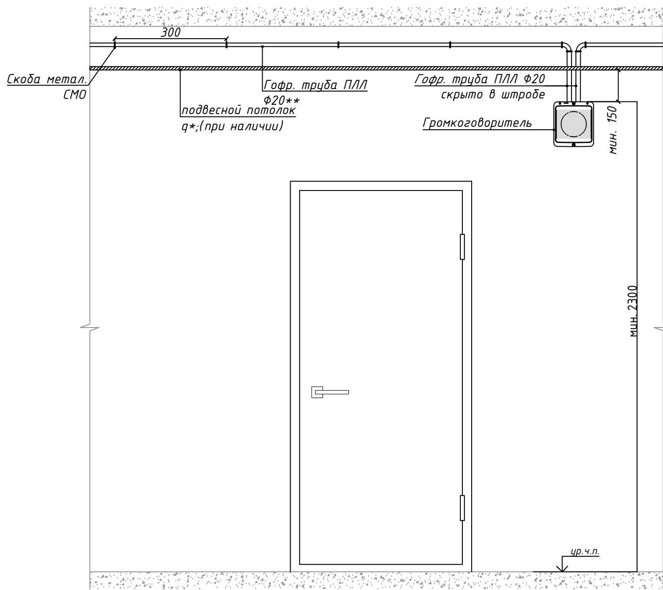
Эскиз установки настенного Громкоговорителя
