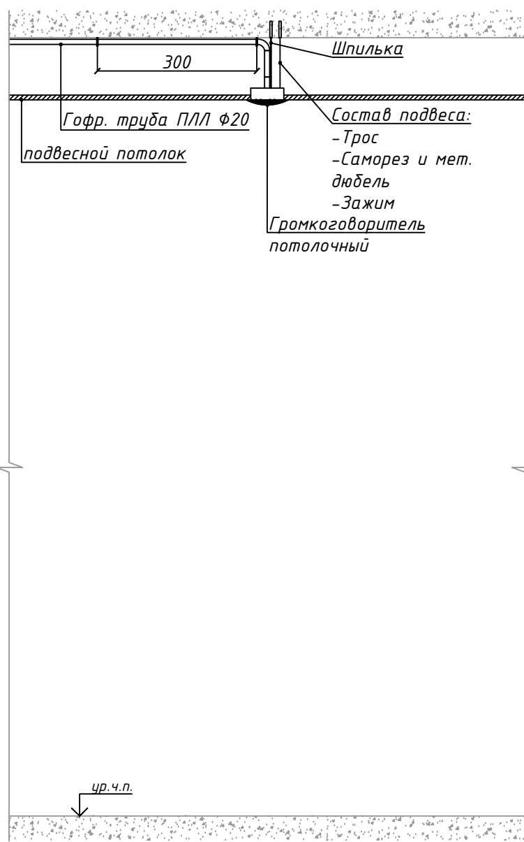
Эскиз установки потолочного Громкоговорителя
