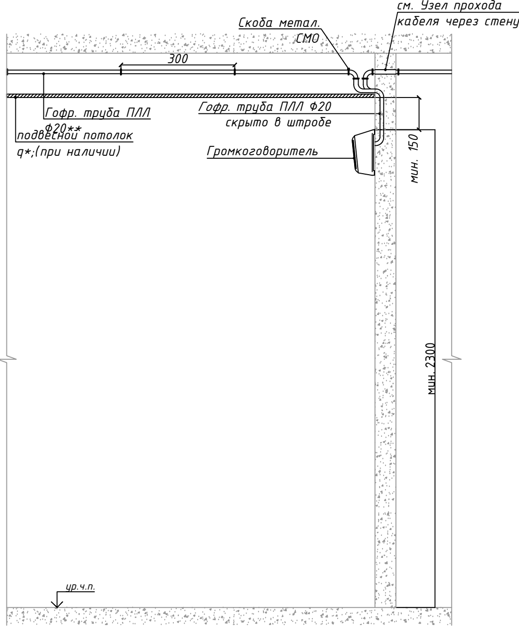
Эскиз установки настенного Громкоговорителя
