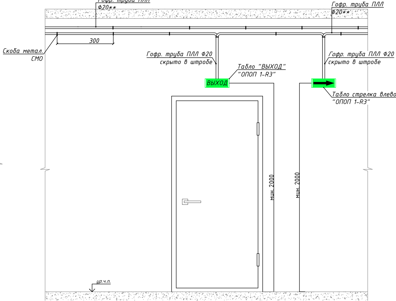
Эскиз установки оборудования на пути эвакуации
